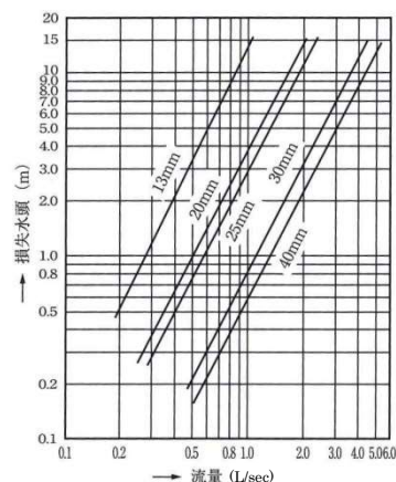
図 2-4 量水器の損失水頭
