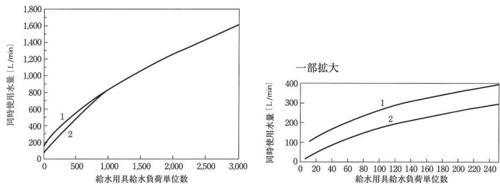
図 2-1 同時使用水量図
