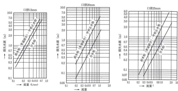
図 2-3 給水栓類の損失水頭（給水栓、止水栓、分水栓）
