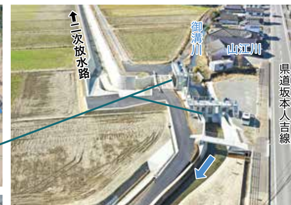
山江川と御溝川の合流地点に水門を設置
