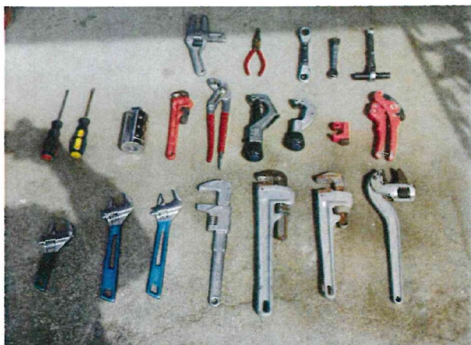
パイプレンチ 350 A L コーナーレンチ イギリス NW280 モンキーレンチ UM25 モンキーレンチ UM36
