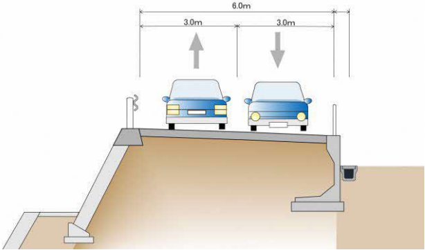
計画幅員（山田川堤防道路線）
