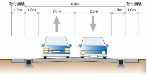
計画幅員（山田川堤防道路線以外）
