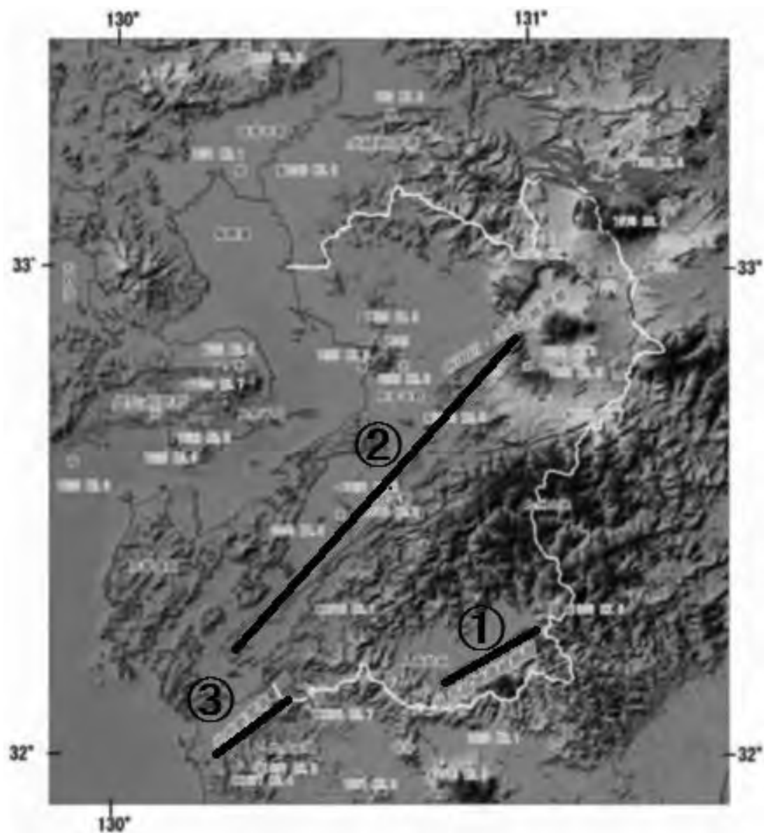
熊本県周辺の主要活断層（図面上の丸数字は前述の想定対象地震）
