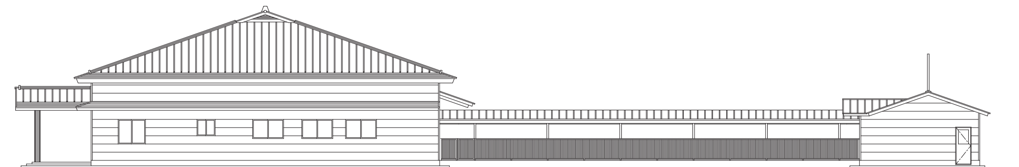
西側立面図 1/150
